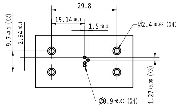
PCB设计示意图 视图比例1:1
